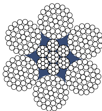
6X37+IWR
