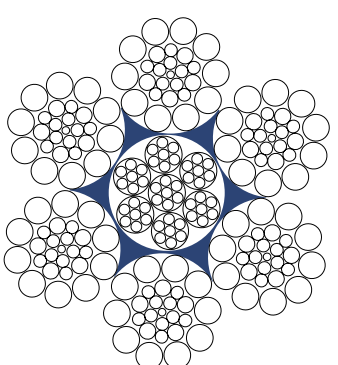
6X26WS+IWR
