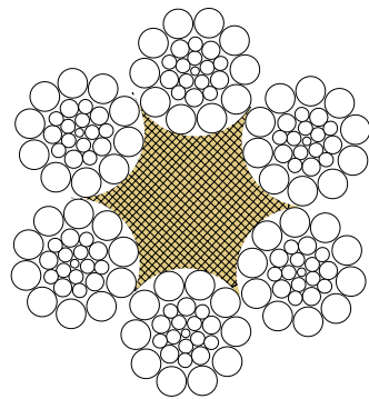
6X26WS+FC
