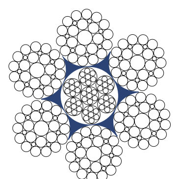
6X29Fi+IWR
