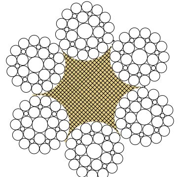
6X29Fi+FC
