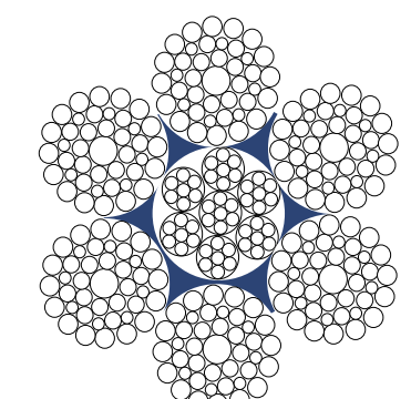
6X41WS+IWR
