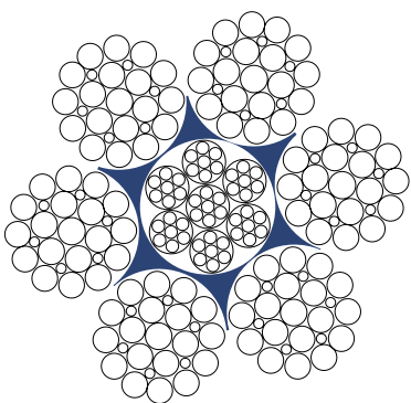
6X25Fi+IWR
