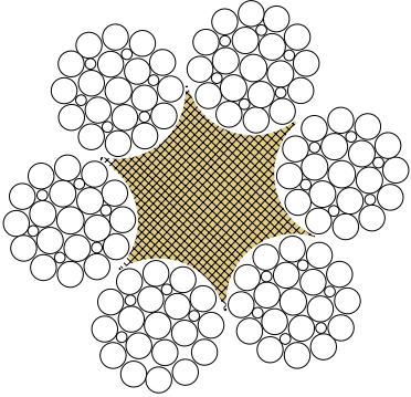
6X25Fi+FC
