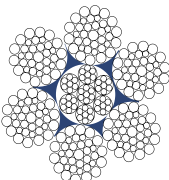
6X36WS+IWR
