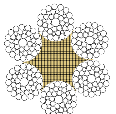
6X41WS+FC
