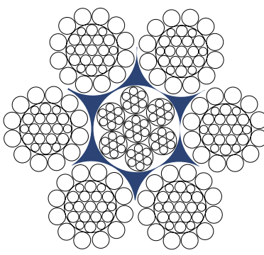
6X31WS+IWR
